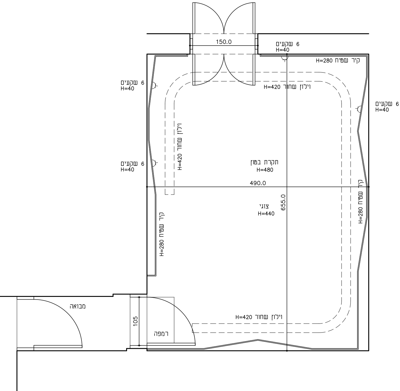
אולפן A קנ"מ 1:50
